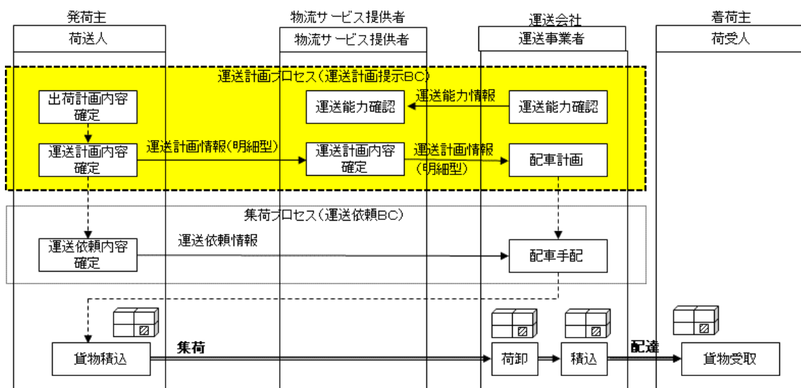
図表A-4 運送計画プロセスのビジネス詳細フロー（物流サービス提供者が参画するケース）
