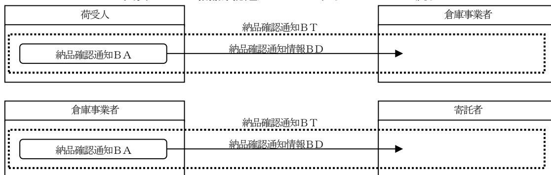
図表R-5 納品確認通知BCのコラボレーションの流れ
