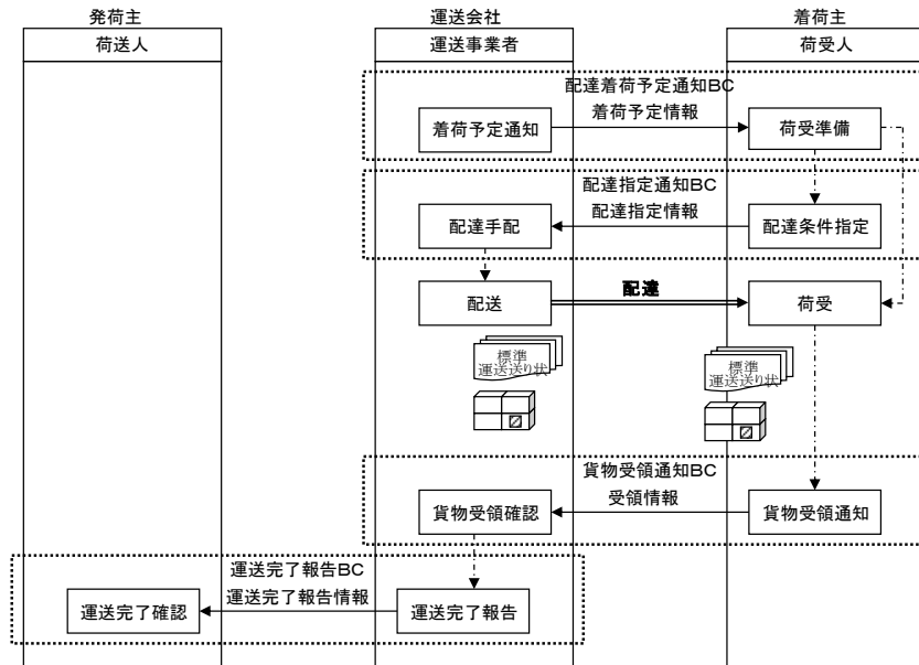
図表C-4 配達プロセスのビジネス詳細フロー（中継運送なし）
